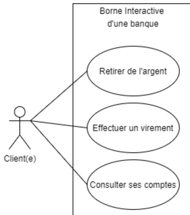
UC : Diagramme des cas d'utilisation d'une borne interactive d'une banque
